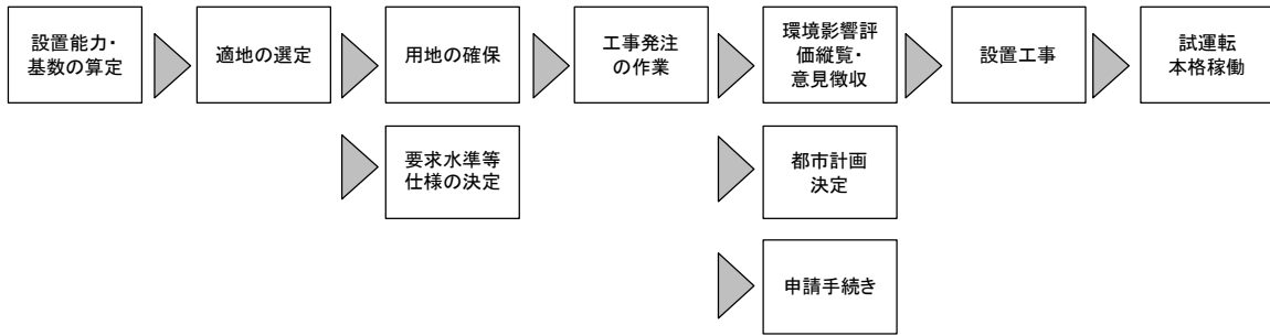
図 7 仮設焼却炉の設置フロー(例)
