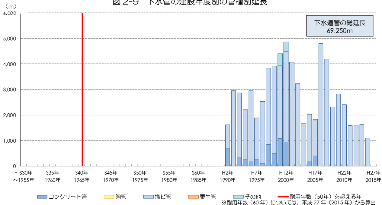
図 2-9 下水管の建設年度別の管種別延長
