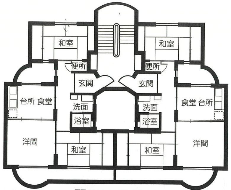
部屋の間取
